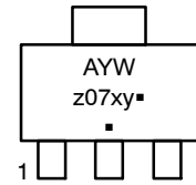
SOT-223 ST SUFFIX CASE 318E
