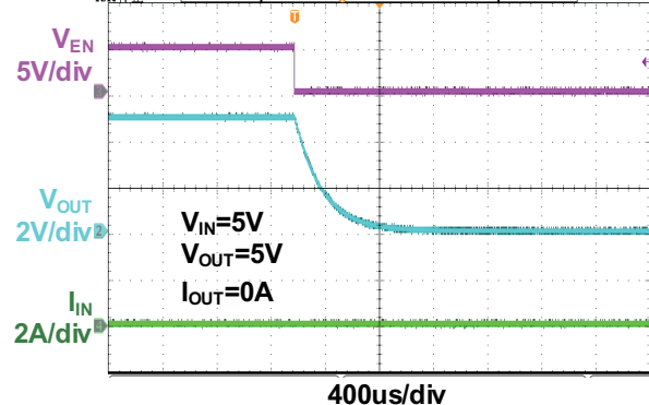
EN Power off ( I_{OUT} = 0A )
