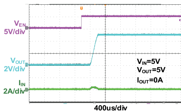
EN Power on ( I_{OUT} = 0A )
